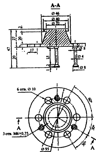
Рисунок 3 — Прибор Красного
