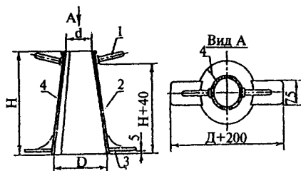
1 – ручка; 2 – корпус; 3 – упоры; 4 – сварной шов.
