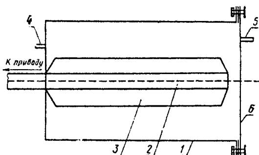
Барабан истирания
