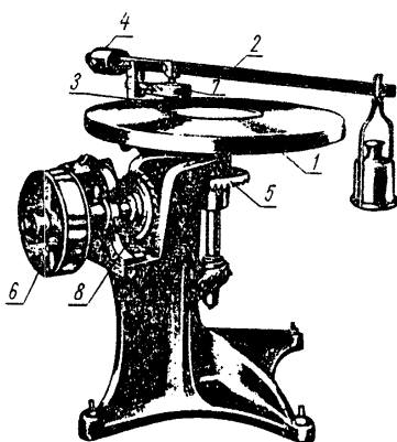
Круг истирания типа Беме
