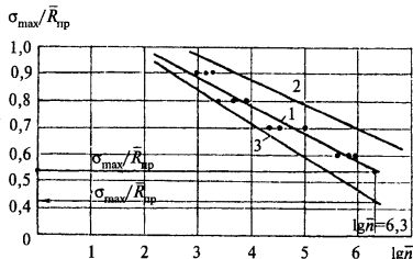
Линия регрессии по результатам испытаний на выносливость
