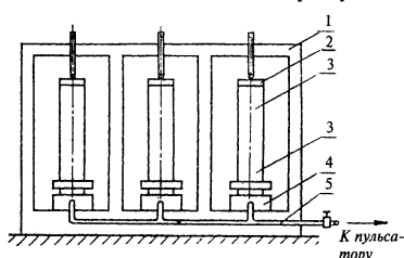
Схема испытательной машины на три образца
