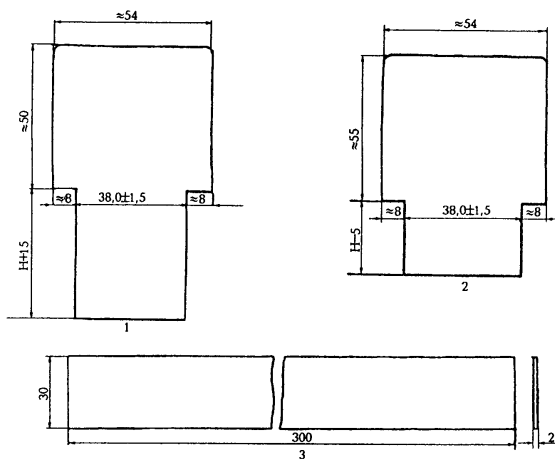
Рисунок 9 — Приспособления для укладки цементного раствора в форму
