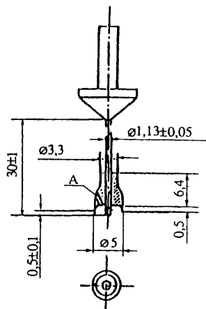
Рисунок 5 — Рабочая часть короткой иглы с кольцеобразной насадкой
