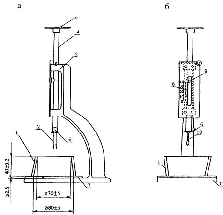
а – положение кольца при определении нормальной густоты и начала схватывания; б – положение кольца при определении конца схватывания 1 – кольцо; 2 – пестик; 3 – пригруз; 4 – цилиндрический металлический стержень; 5 – обойма станины; 6 – стопорное устройство; 7 – пластинка; 8 – шкала; 9 – указатель; 10 – игла; 11 – основание станины
