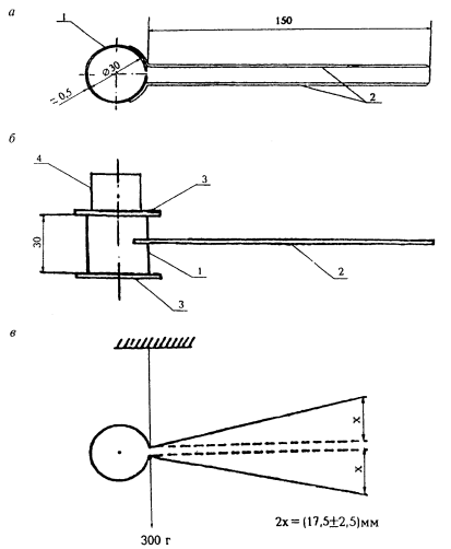
a – кольцо Ле Шателье (вид сверху); б – кольцо Ле Шателье с пластинками и пригрузом (вид сверху); в – схема поверхности упругости кольца Ле Шателье 1 – кольцо с прорезью; 2 – индикаторная игла; 3 – пластинка; 4 – пригруз Рисунок 7
