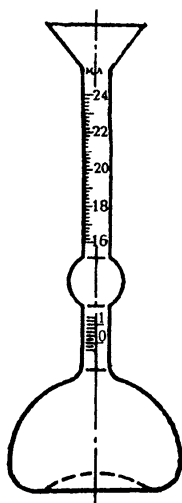
Рисунок 1 — Прибор Ле Шателье
