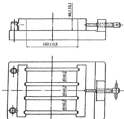
Рисунок 8 — Форма для изготовления образцов-балочек
