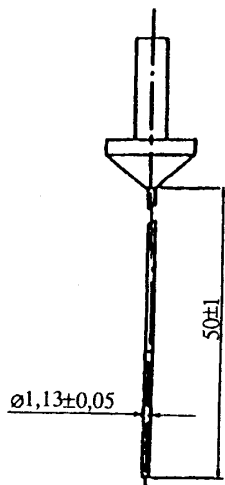
Рисунок 4 – Рабочая часть длинной иглы
