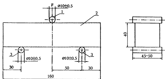
Рисунок 10 — Схема расположения образца-балочки при испытании на изгиб
