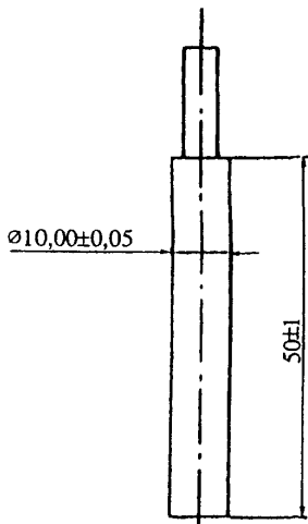
Рисунок 3 – Рабочая часть пестика
