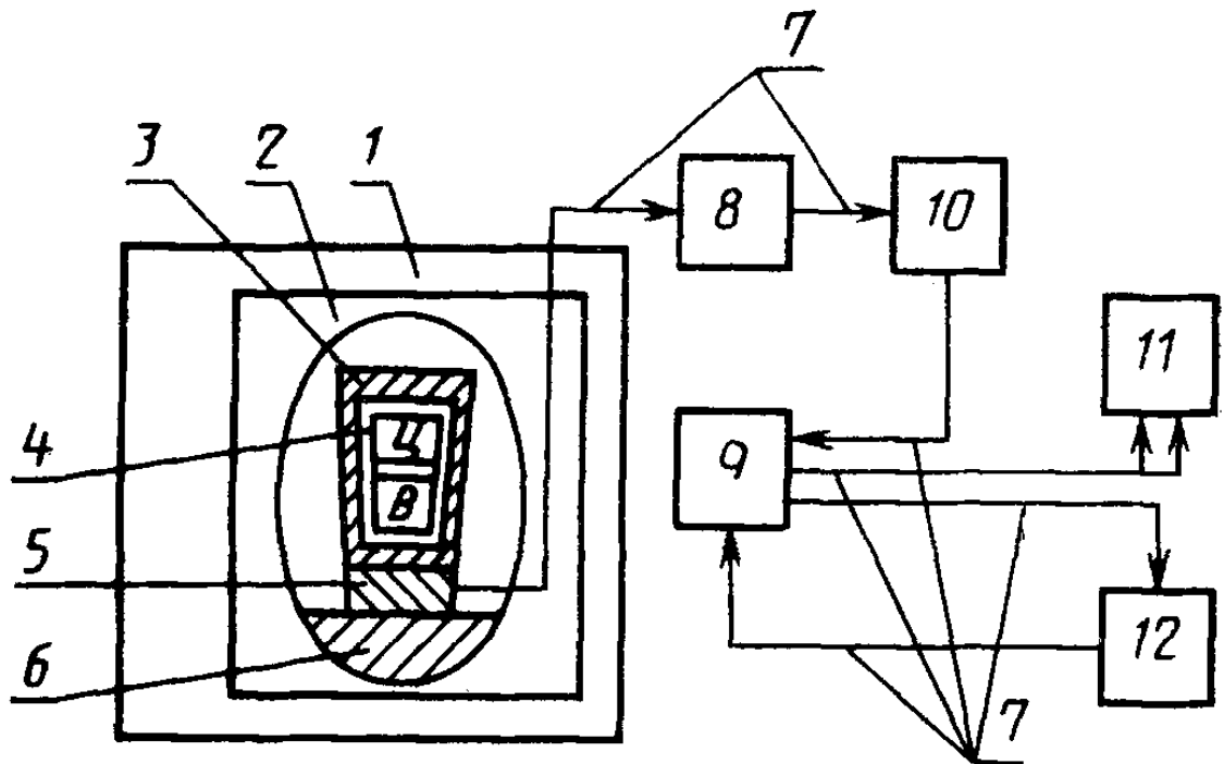
1 — термостат; 2 — калориметрический блок; 3 — камера; 4 — ячейка; 5 — термомер; 6 — теплоотвод; 7 — соединительные кабели; 8 — коммутатор; 9 — калибратор; 10 — предварительный усилитель; 11 — самописец; 12 — интегратор
