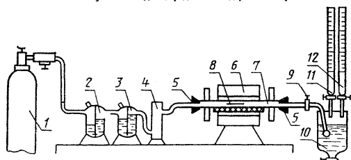
Схема установки для определения содержания серы
