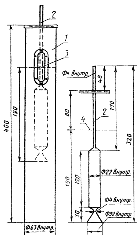
1 — цилиндр; 2 — пипетка; 3 — метка (1000 мл); 4 — уровень суспензии в цилиндре Черт. 3
